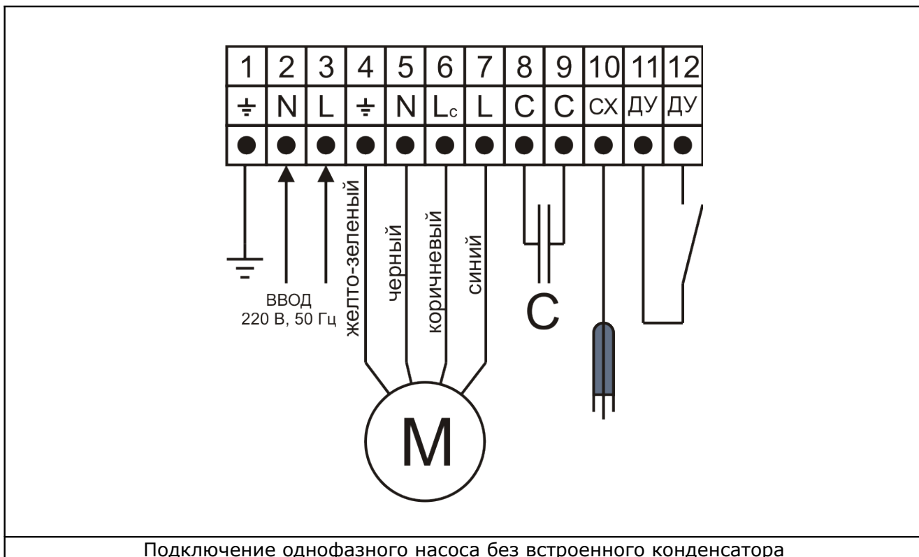
Рис.1 - Электроподключение
